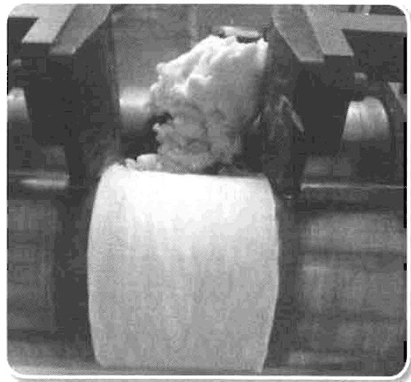
รูปที่ 1 บดผสมยางกับกำมะถัน ด้วยเครื่องบดผสมแบบ 2 ลูกกลิ้ง (Two-rolls mill)
